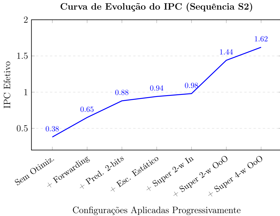
Figura 4: Curva de ganho incremental de IPC na sequência de loop S2 com base nas otimizações arquiteturais e estáticas.
