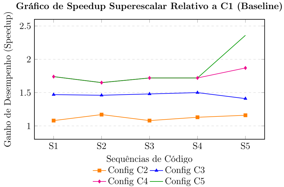
Figura 3: Curvas de aceleração obtidas pelas arquiteturas especulativas e OoO em relação ao baseline superescalar rígido (C1).
