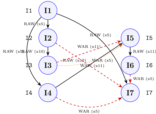
Figura 2: Grafo Otimizado de Dependências de Dados e Restrições de Nomes — Sequência S4.
